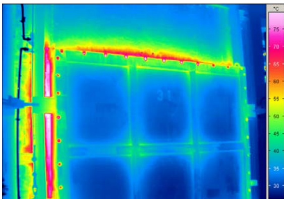
Furnace door
