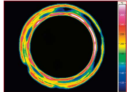
Darstellung einer Rotationsprüfung im Thermografenbild
