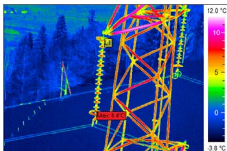
Wärmebild eines Hochspannungsmast
