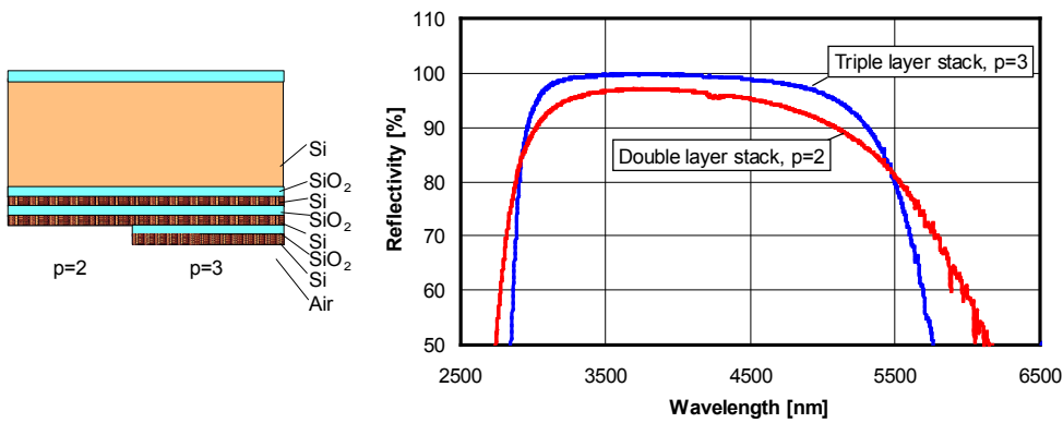
Bild 6 Gemessener spektraler Reflektionsgrad von Bragg-Reflektoren (relativ zu Au-Standard)
